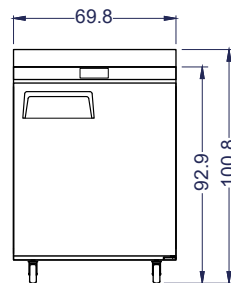
MGF8412-MFR27"
