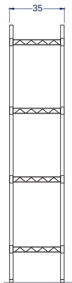
Vista Izquierda
