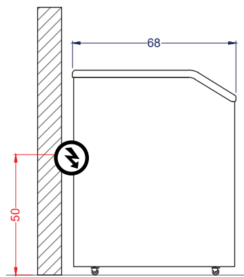
Vista Izquierda
